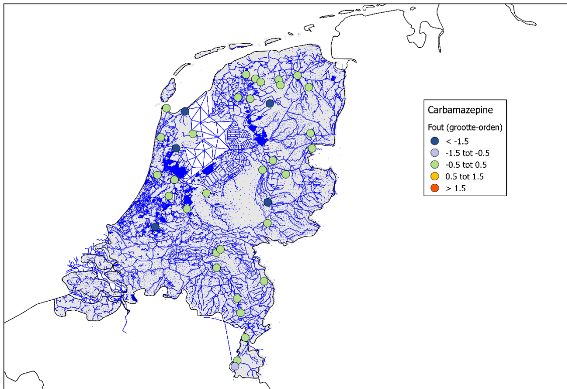
Figuur 4.16 De fout per station ( N = 37 ) voor carbamazepine, afgebeeld in een correlatiegrafiek en een kaart. Merk op dat drie stations met fouten van -8, -14 en -15 omwille van de leesbaarheid niet zijn afgebeeld in de grafiek.
