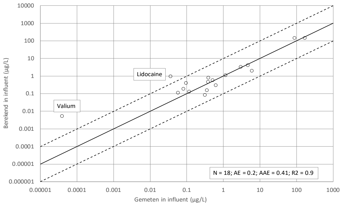
Figuur 2.5 Best mogelijk geschatte concentratie in influent uitgezet tegen de waargenomen concentratie in influent; gebruiksvolumen gebaseerd op werkelijke data, excretiefactor van Oldenkamp et al. (2018).
