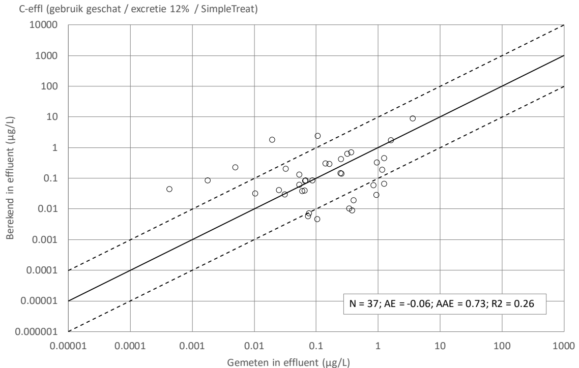
Figuur 2.8 Geschatte concentratie in effluent uitgezet tegen de waargenomen concentratie in effluent; gebruiksvolumen geëxtrapoleerd op basis van data uit VK en Zweden, homogene excretiefactor van 12%, zuiveringsrendement uit SimpleTreat.
