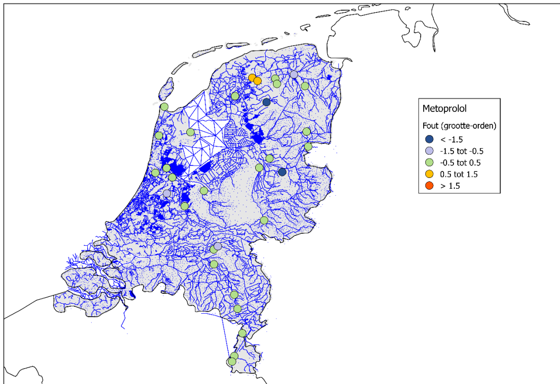
Figuur 4.17 De fout per station ( N = 31 ) voor metoprolol, afgebeeld in een correlatiegrafiek en een kaart. Merk op dat een station met een fout van -11 omwille van de leesbaarheid niet is afgebeeld in de grafiek.
