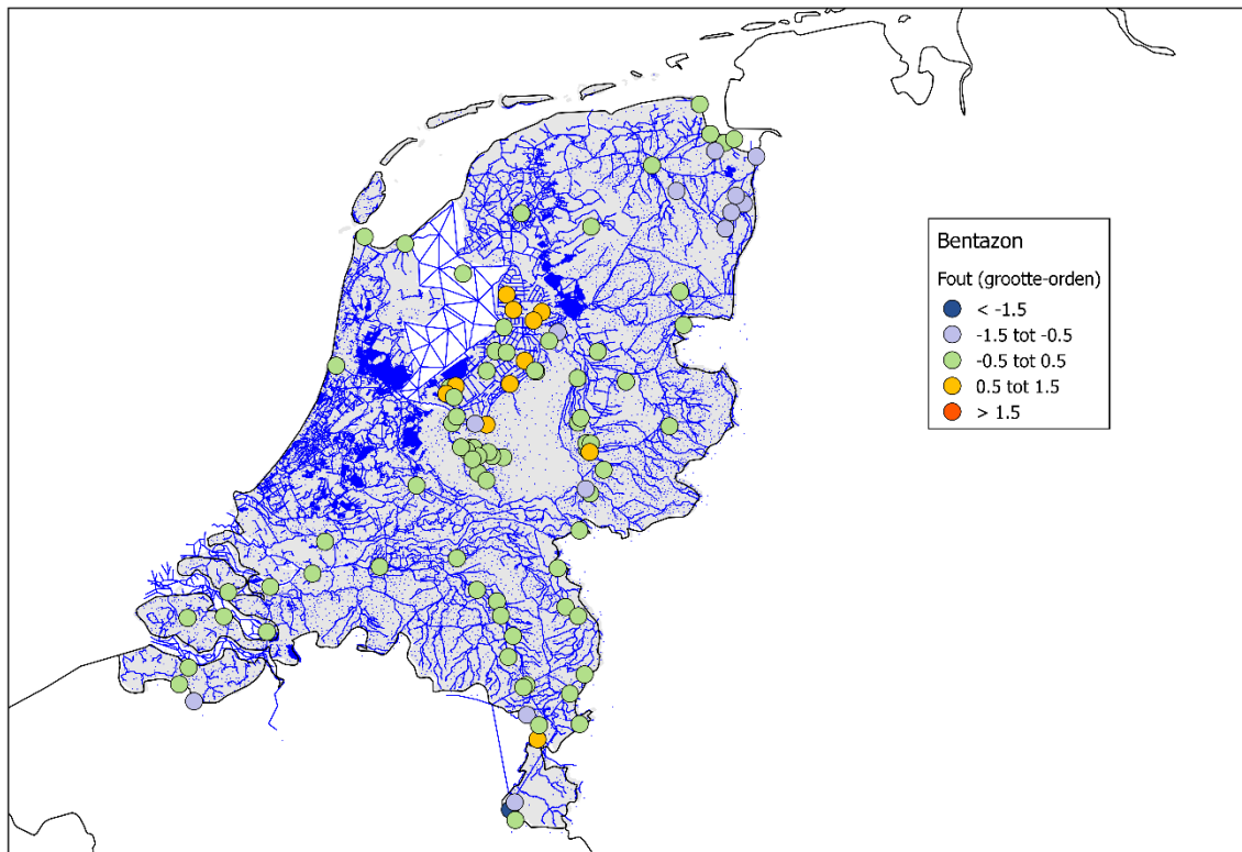
Figuur 4.19 De fout per station ( N = 99 ) voor bentazon, afgebeeld in een correlatiegrafiek en een kaart.
